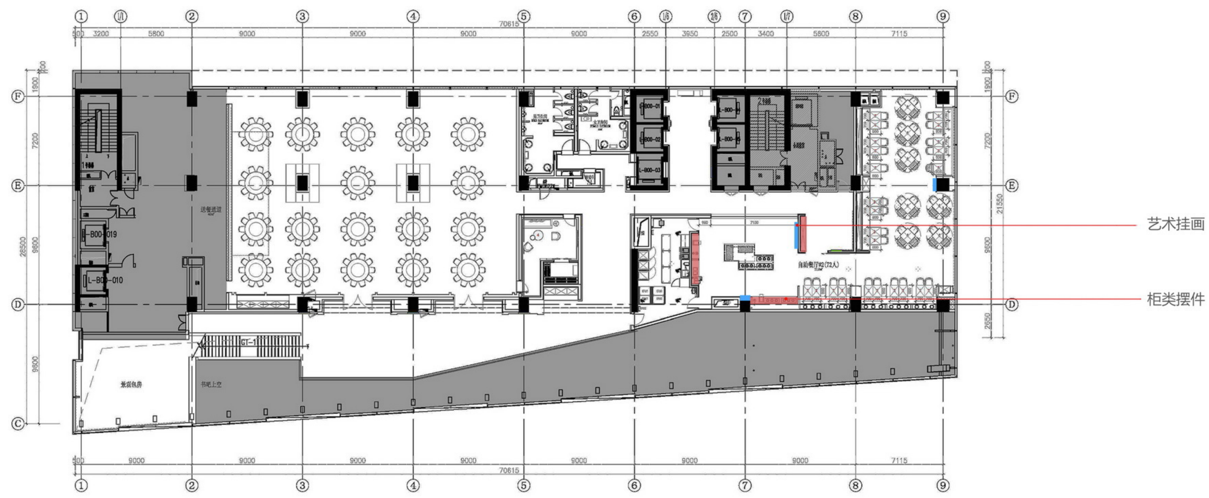
六层平面图
